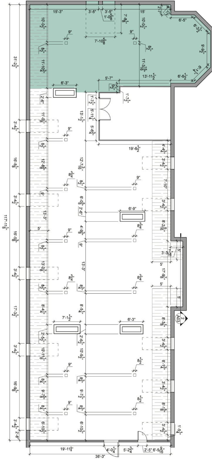
1 PLAN DE LA GALERIE ECHELLE: \frac{1}{8}'' = 1' - 0''
